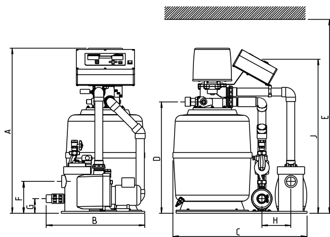
Abb. 2 Maßzeichnung Filteranlage GENO-mat® F 500 AK
